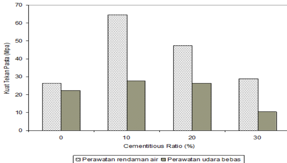
Gambar 3 Grafik hubungan kuat tekan pasta dengan metode perawatan
