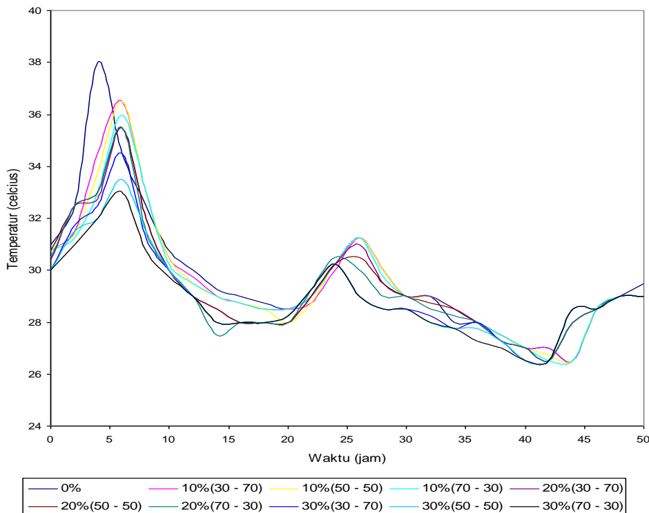
Gambar 2 Grafik Temperatur Hidrasi
