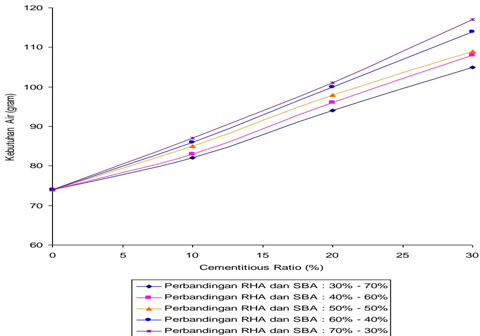
Gambar 1 Grafik Hubungan C R dan Berat Air
