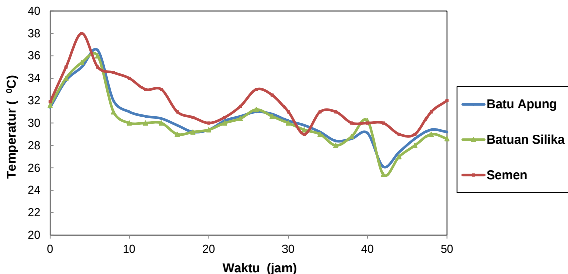
Gambar 1 Perkembangan temperatur hidrasi pasta semen selama 50 jam
