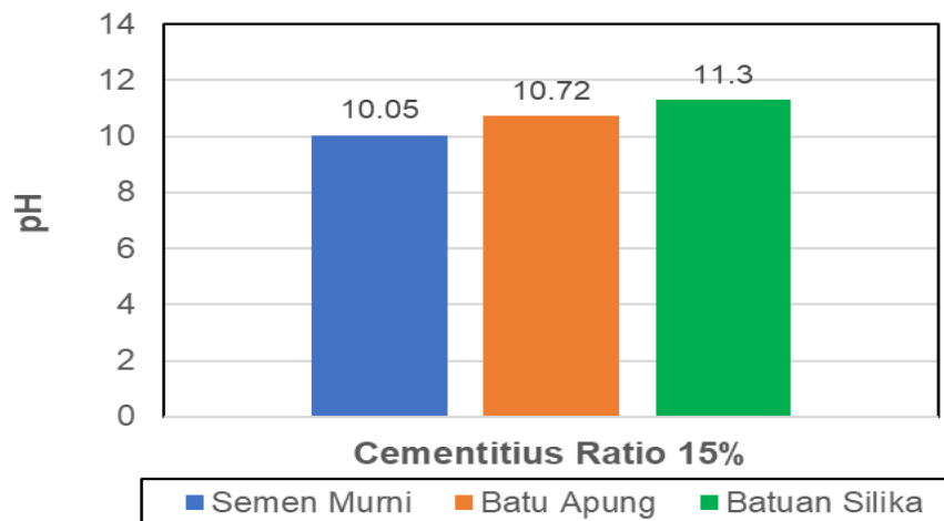
Gambar 4 Grafik Hubungan CR – pH
