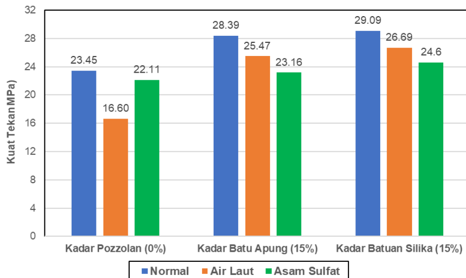
Gambar 3 Grafik Hubungan Kuat Tekan Mortar Umur 90 Hari
