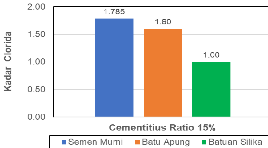
Gambar 5 Grafik Hubungan CR – Kadar Clorida
