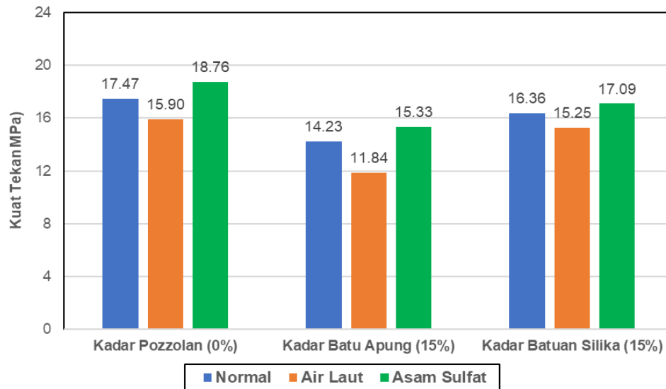
Gambar 2 Grafik Hubungan Kuat Tekan Mortar Umur 28 Hari
